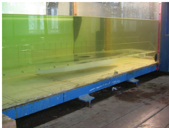
Рис. 3. Розташування пластини з овальною лункою у вимірювальному участку гідродинамічного лотку
