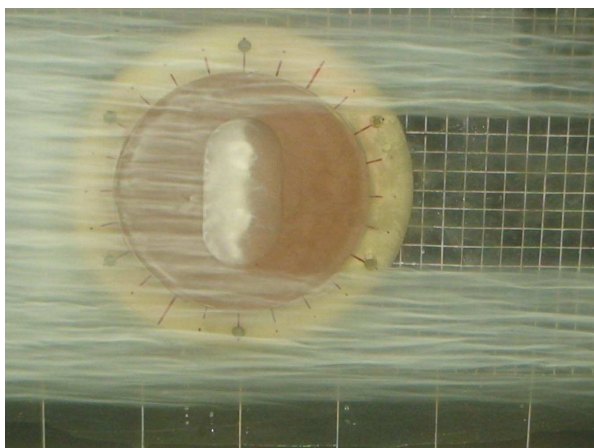
Рис. 8. Синхронний викид когерентних великомасштабних вихорів із трьох областей овальної лунки при швидкості течії 0.25 м/с
