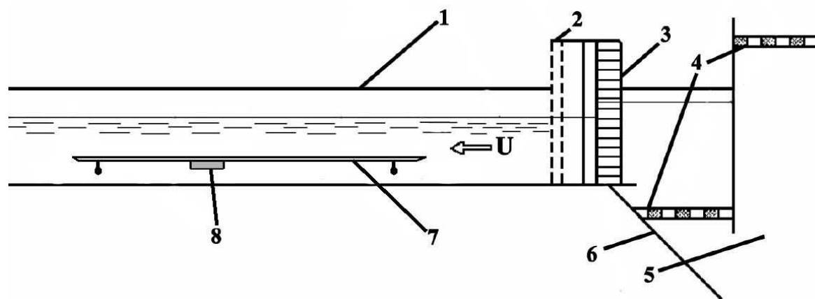
Рис. 1. Схема експериментальної установки: 1 – гідродинамічний лоток, 2 – сітки, 3 – хонейкомб, 4 – решітки, 5 – заспокійлива камера, 6 – конфузор, 7 – пластина, 8 – овальна лунка
