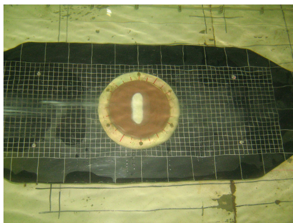
Рис. 9. Формування веретеноподібного вихору усередині поперечно обтічної овальної лунки при швидкості течії 0.5 м/с
