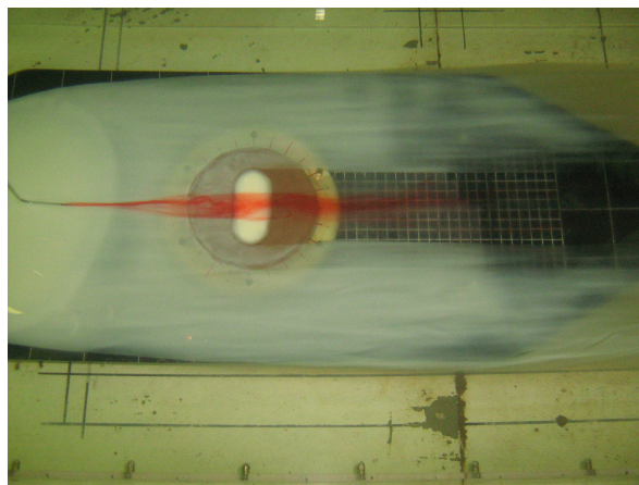
Рис. 5. Взаємодія набігаючого потоку з рідиною усередині овальної лунки при швидкості течії 0.1 м/с
